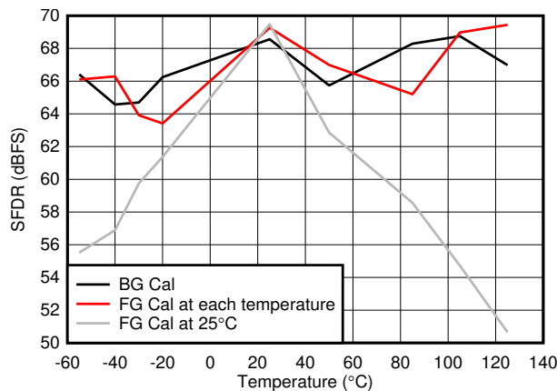
图 7-65. SFDR vs Temperature
