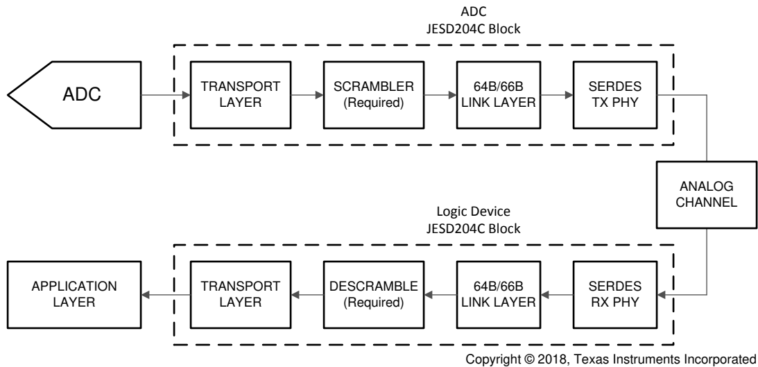
图 8-6. Simplified 64B/66B Encoded JESD204C Interface Diagram
