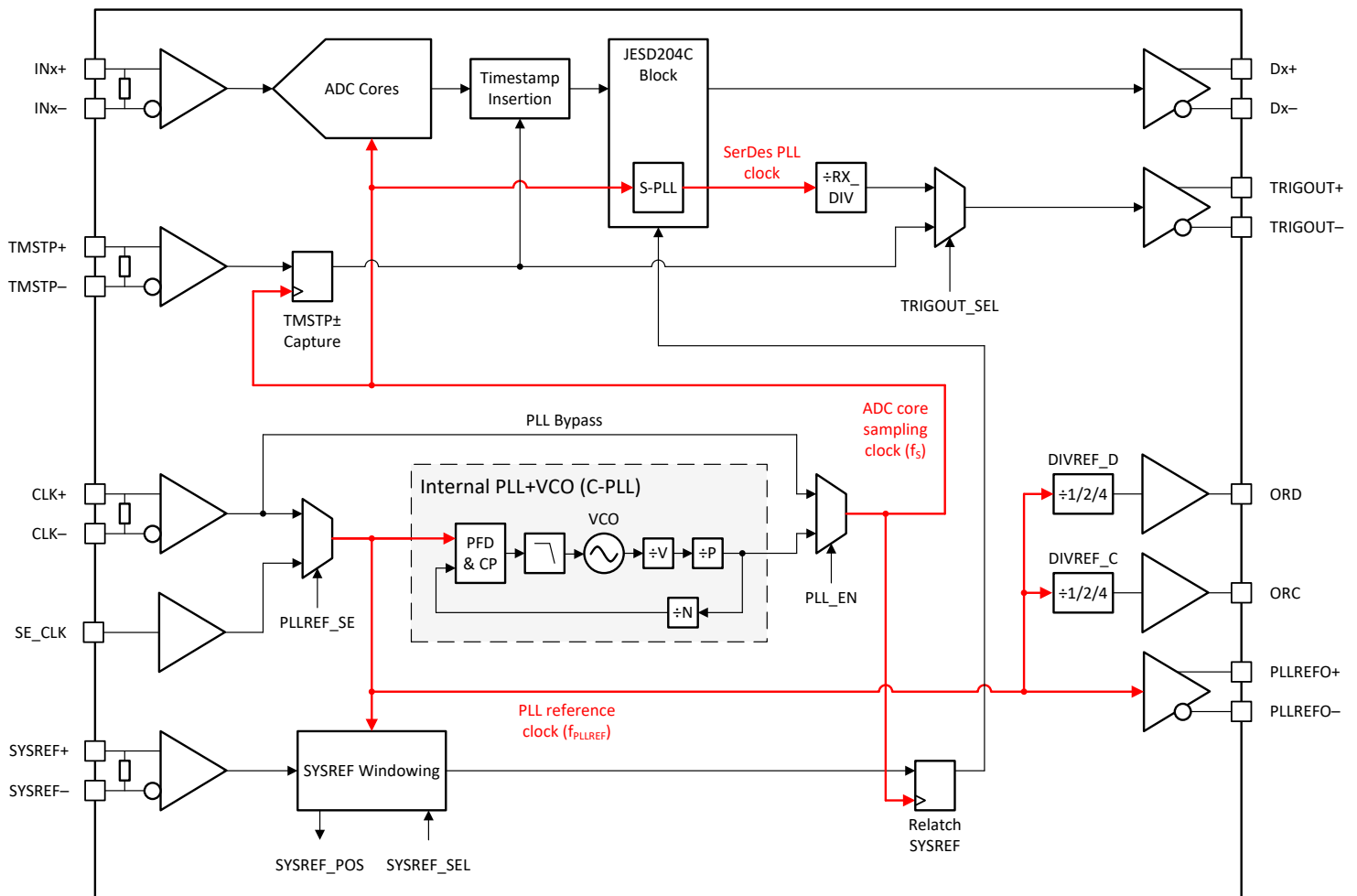
图 8-3. Clocking Subsystem
