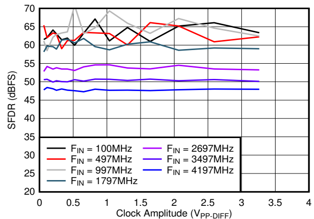
图 7-36. SFDR vs A_{CLK}
