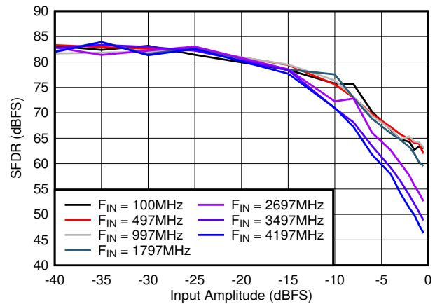
图 7-32. SFDR vs A_{IN}
