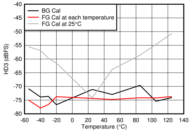
图 7-67. HD3 vs Temperature
