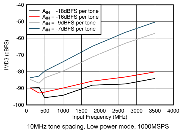
图 7-76. IMD3 vs F_{IN}
