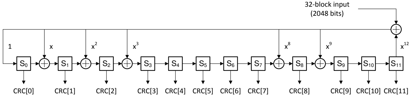
图 8-7. CRC-12 Parity Bit Generator
