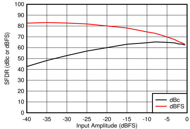
图 7-32. SFDR vs A_{IN}
