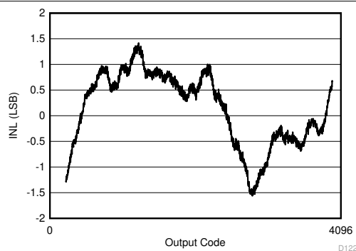
图 7-2. INL vs Code
