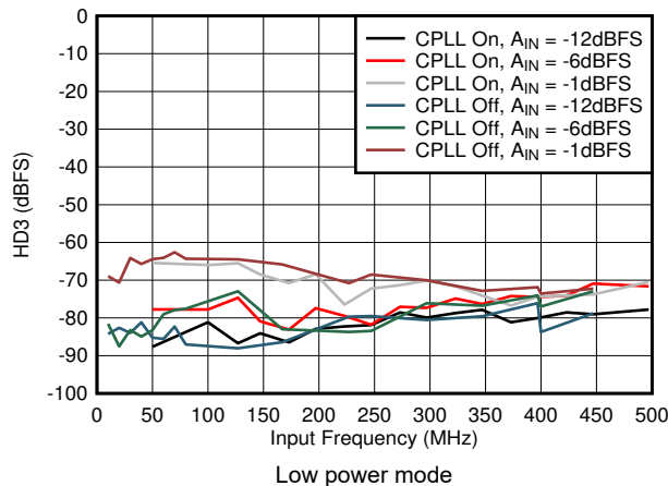
图 7-59. HD3 vs A_{IN} and C-PLL
