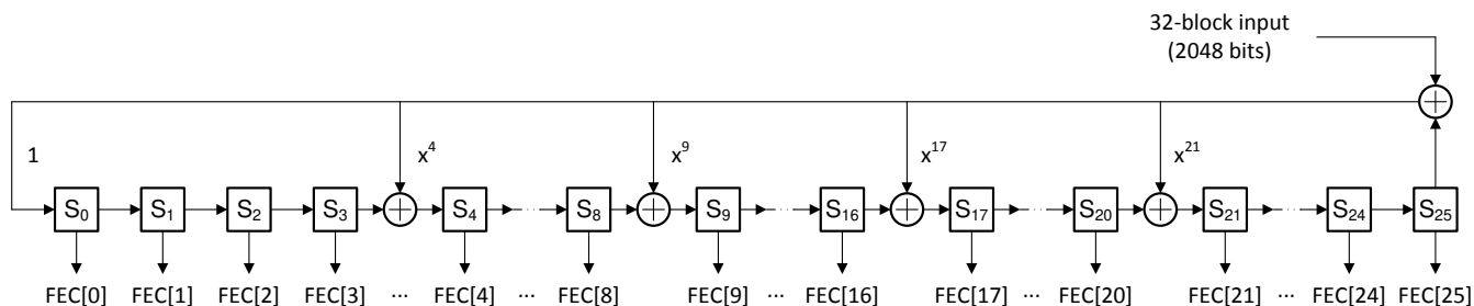
图 8-8. FEC Parity Bit Generator
