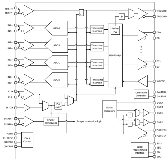
四通道器件方框图
