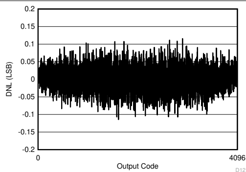
图 7-1. DNL vs Code
