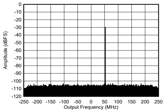
图 6-214. RX Output FFT at 6.851 GHz and -30 dBFS
