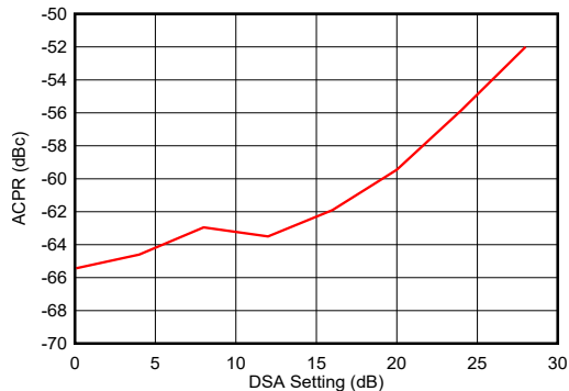
图 6-333. TX 20-MHz LTE ACPR vs DSA at 0.85 GHz
