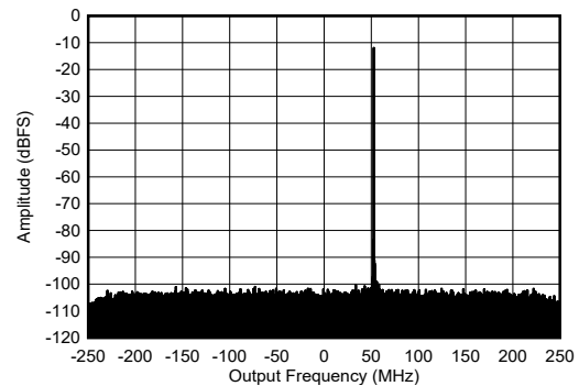
图 6-213. RX Output FFT at 6.851 GHz and -12 dBFS
