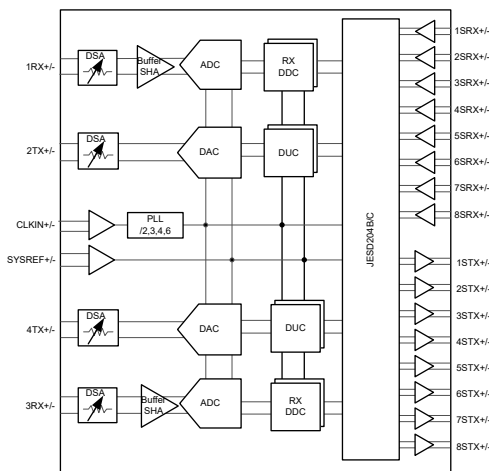
功能方框图
