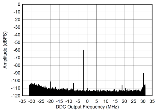
图 6-17. RX Output FFT at 30 MHz
