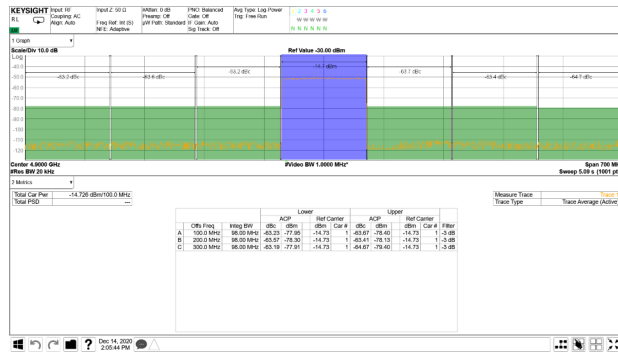
图 6-526. TX 100-MHz NR Output Spectrum at 4.9 GHz
