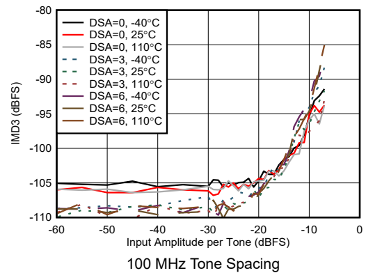
图 6-217. RX IMD3 vs Input Amplitude at 6.851 GHz
