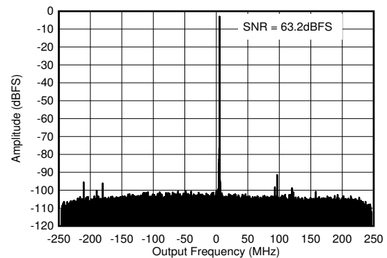
图 6-61. RX Output FFT at 0.8 GHz
