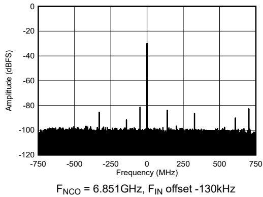
图 6-214. RX Output FFT at 6.851GHz and -30dBFS
