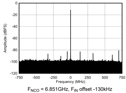
图 6-213. RX Output FFT at 6.851GHz and -12dBFS
