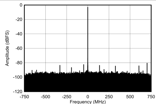
图 6-211. RX Output FFT at 6.851GHz and -3dBFS
