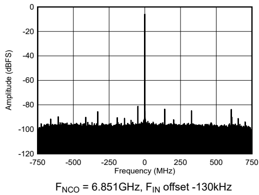
图 6-212. RX Output FFT at 6.851GHz and -6dBFS
