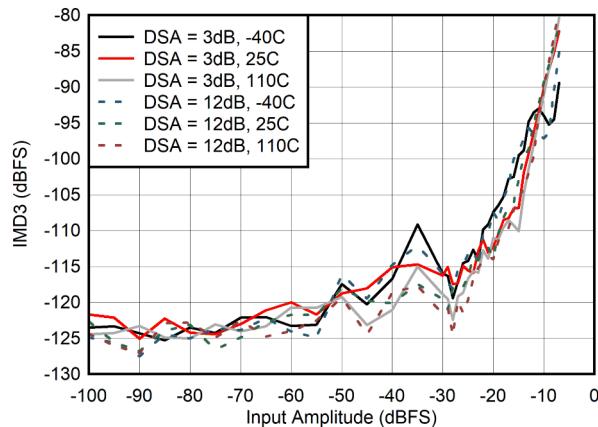
图 6-45. IMD3 vs Input Amplitude at 400MHz
