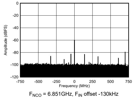
图 6-215. RX Output FFT at 6.851GHz and -60dBFS
