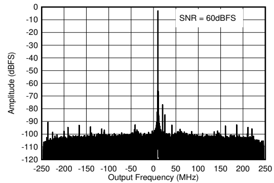
图 6-184. RX Output FFT at 4.9 GHz
