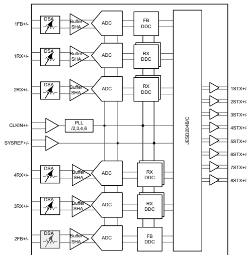
功能方框图
