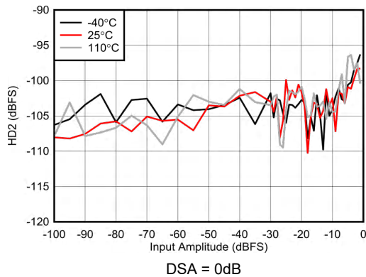
图 6-222. RX HD2 vs Input Amplitude at 6.851GHz
