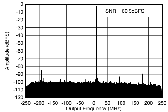
图 6-92. RX Output FFT at 1.75 GHz
