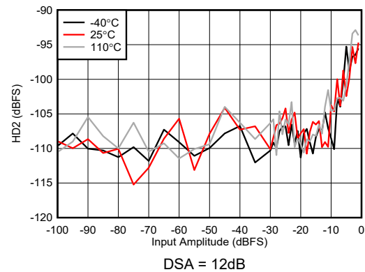
图 6-223. RX HD2 vs Input Amplitude at 6.851GHz
