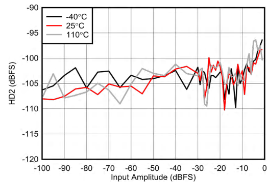
图 6-221. RX HD2 vs Input Amplitude at 6.851GHz
