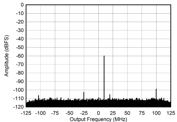
图 6-42. RX Output FFT at 405 MHz and -60dBFS
