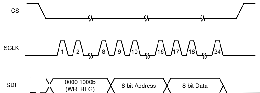
图 7-9. Register Write Operation
