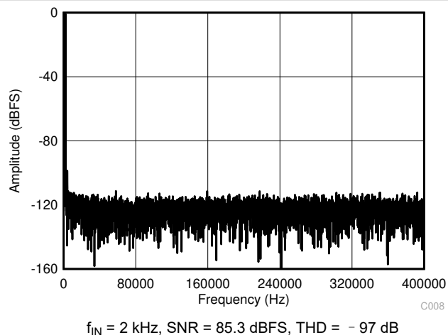
图 6-14. Typical FFT
