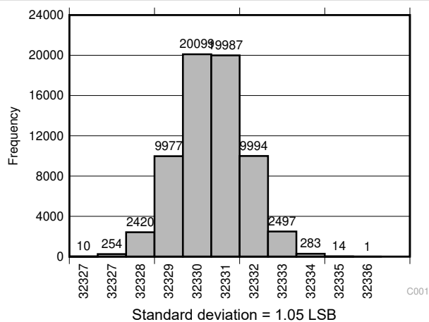
图 6-13. DC Input Histogram
