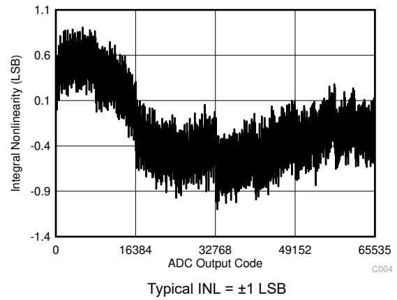
图 6-4. Typical INL
