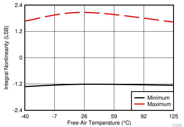
图 6-4. Typical INL
