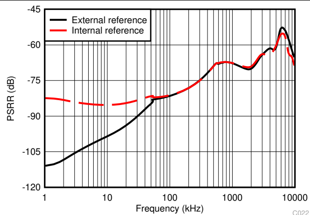
图 6-22. PSRR vs Frequency
