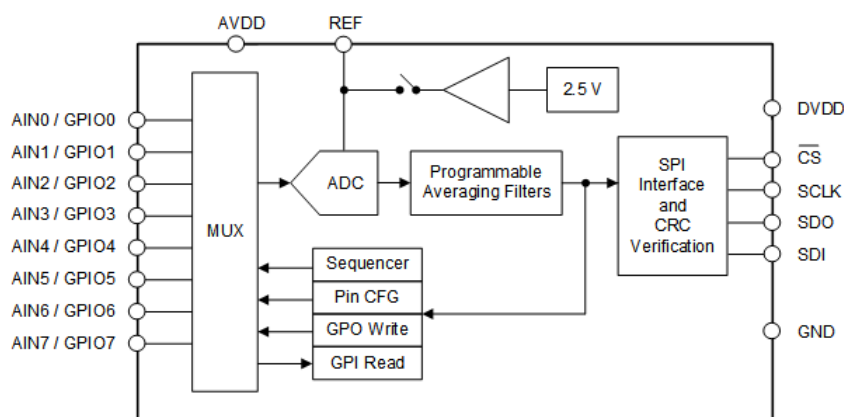
ADS7067 方框图
