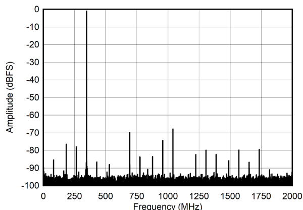
图 8-3. FFT for 347 MHz Input Signal, 4 GSPS, JMODE3
