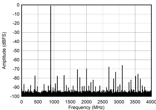
图 6-9. DES Mode: Single Tone FFT at 897 MHz
