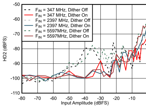
图 6-60. DES Mode: HD2 vs Input Amplitude and Dither
