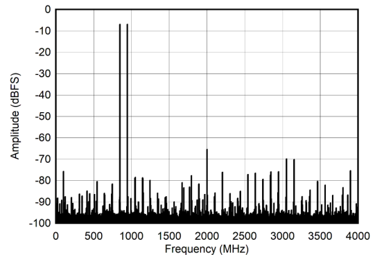
图 6-14. DES Mode: Two Tone FFT at 897 MHz
