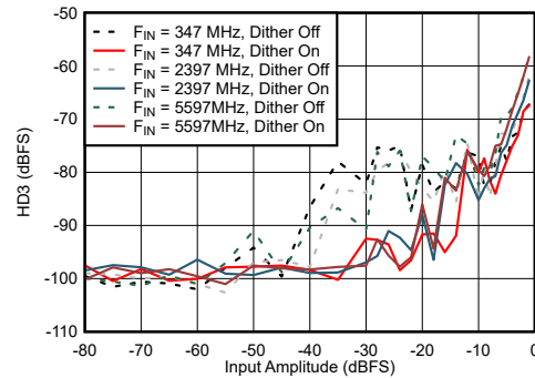
图 6-62. DES Mode: HD3 vs Input Amplitude and Dither
