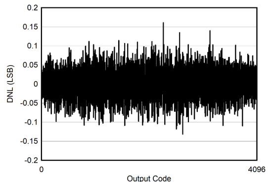
图 6-6. DNL vs ADC Code
