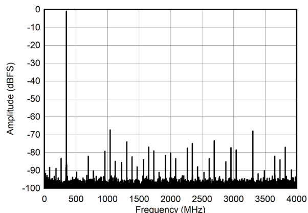
图 8-2. FFT for 347 MHz Input Signal, 8 GSPS, JMODE1
