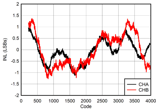
图 6-7. INL vs ADC Code
