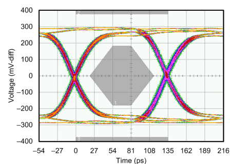
7.4Gb/s 时的输出串行信道眼图
