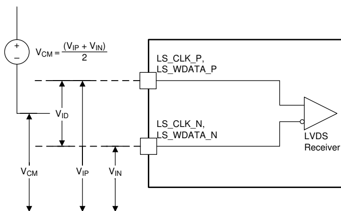
图 5-7. LSIF 电压要求
