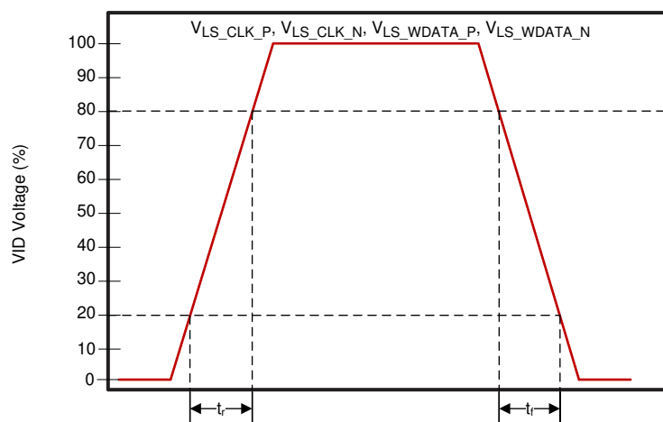
图 5-6. LSIF 上升/下降时间压摆率
