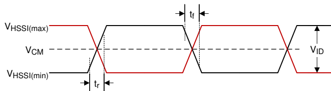
图 5-11. HSSI 波形要求
