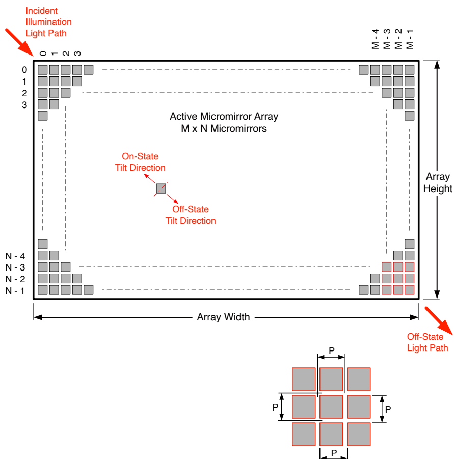
图 5-15. 微镜阵列物理特性
