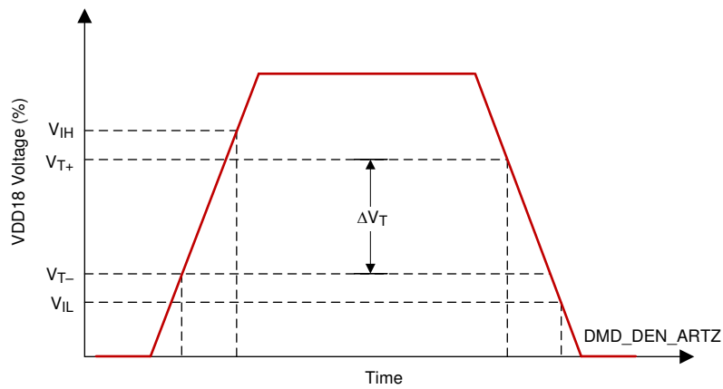
图 5-9. LVC MOS 输入迟滞
