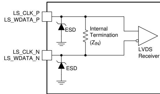
图 5-8. LSIF 等效输入
