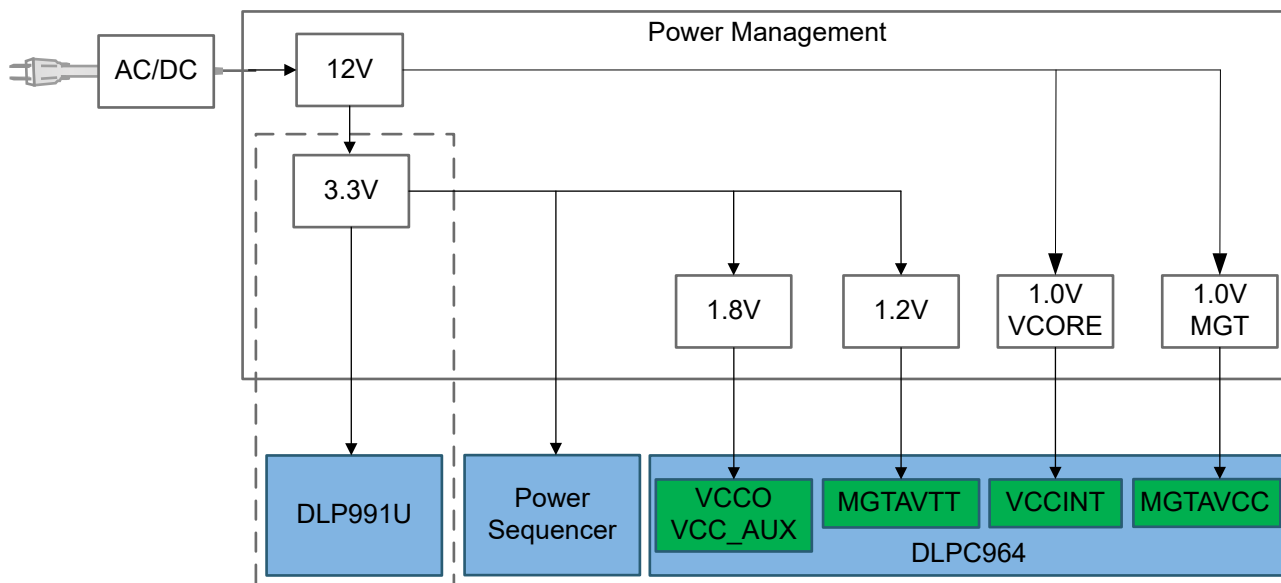
图 7-11. Power Distribution
