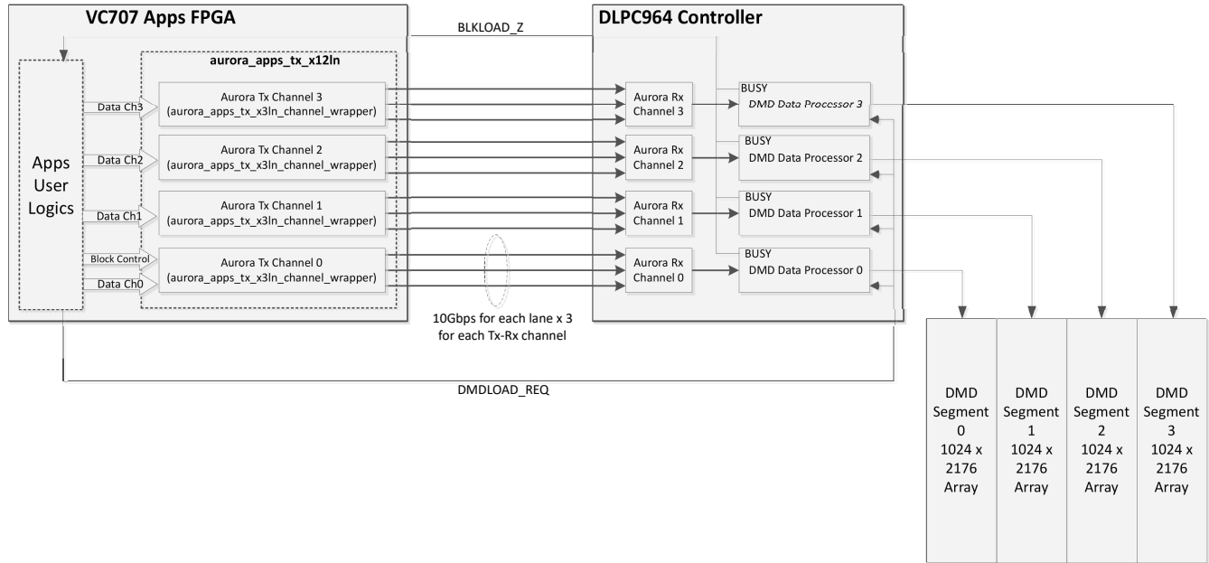
图 7-3. DLPC964 System Block Diagram
