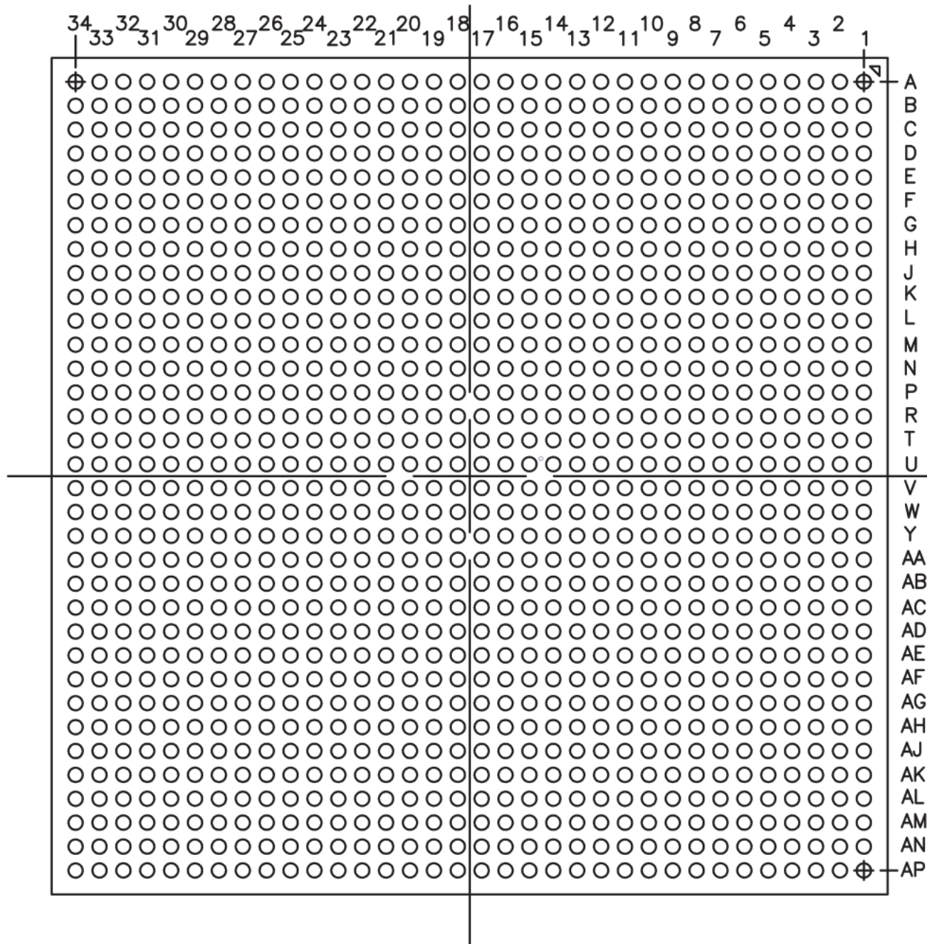
图 4-1. ZUM Package, 1158-Pin FCBGA, Bottom View
