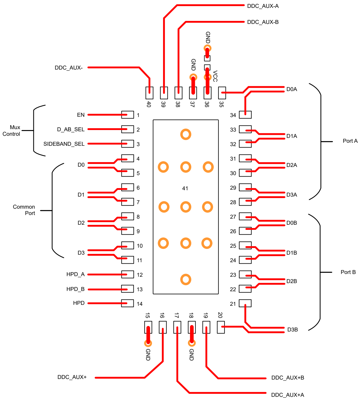
图 8-2. 布局示例
