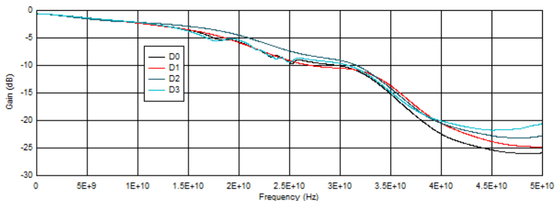
图 5-2. 端口 B 的差分插入损耗与频率间的关系
