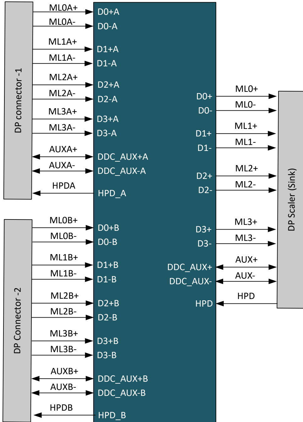
图 8-3. DisplayPort 2:1 开关
