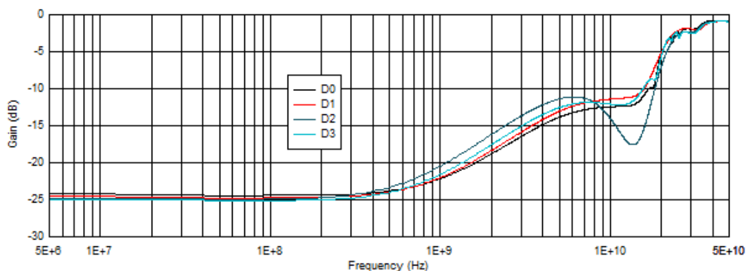
图 5-3. 选择端口 A 时的输入差分回波损耗特性
