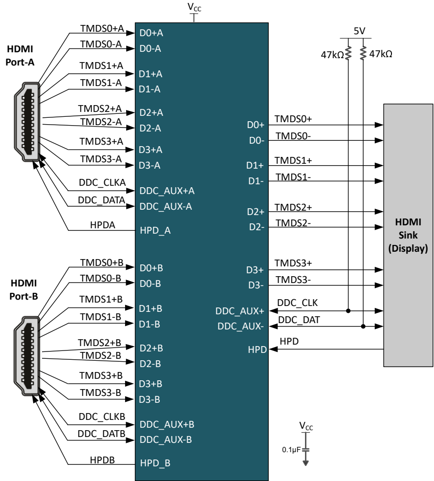
图 8-1. 选择两个 HDMI 端口之一 - 应用原理图
