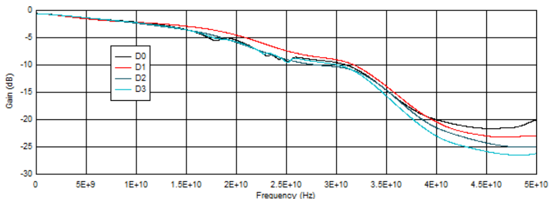
图 5-1. 端口 A 的差分插入损耗与频率间的关系
