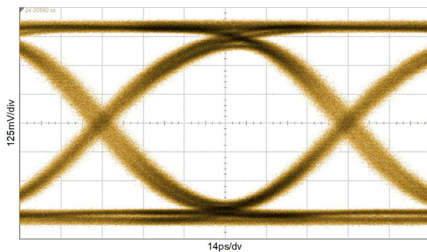
图 7-12. OUT0± 为 11.88Gbps (12G-SDI), CC = 100m Belden 1694A 位于 SDI_IN+, 经过时钟恢复
