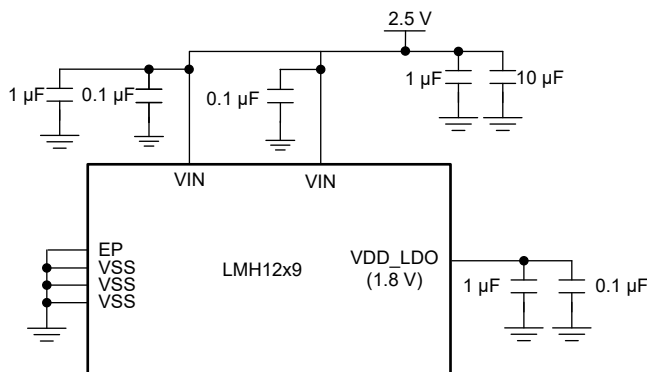
图 7-18. 建议的电源去耦
