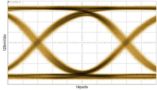
图 5-2. 在 OUT1± 上测得，100m Belden 1694A，SDI_IN+ 前，禁用 SDI_OUT
