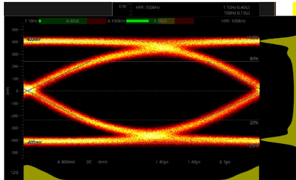
图 5-3. 在 SDI_OUT+ 上测得，1m Belden 1694A 后
