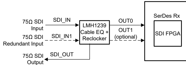
图 7-10. LMH1239 具有冗余 SDI 输入的电缆均衡器应用
