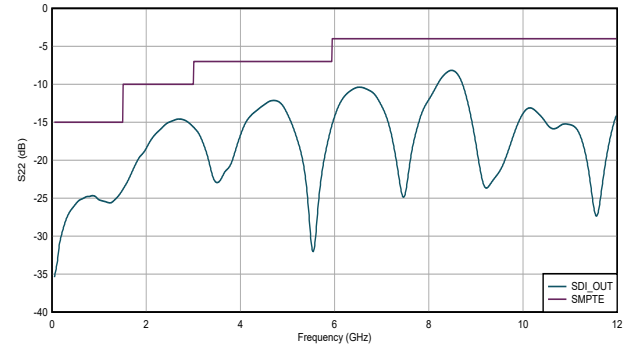
图 5-4. 输出回波损耗 (RL) 与频率间的关系
