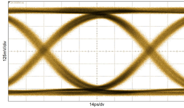
图 5-1. 在 OUT0± 上测得，100m Belden 1694A，SDI_IN+ 前，禁用 SDI_OUT
