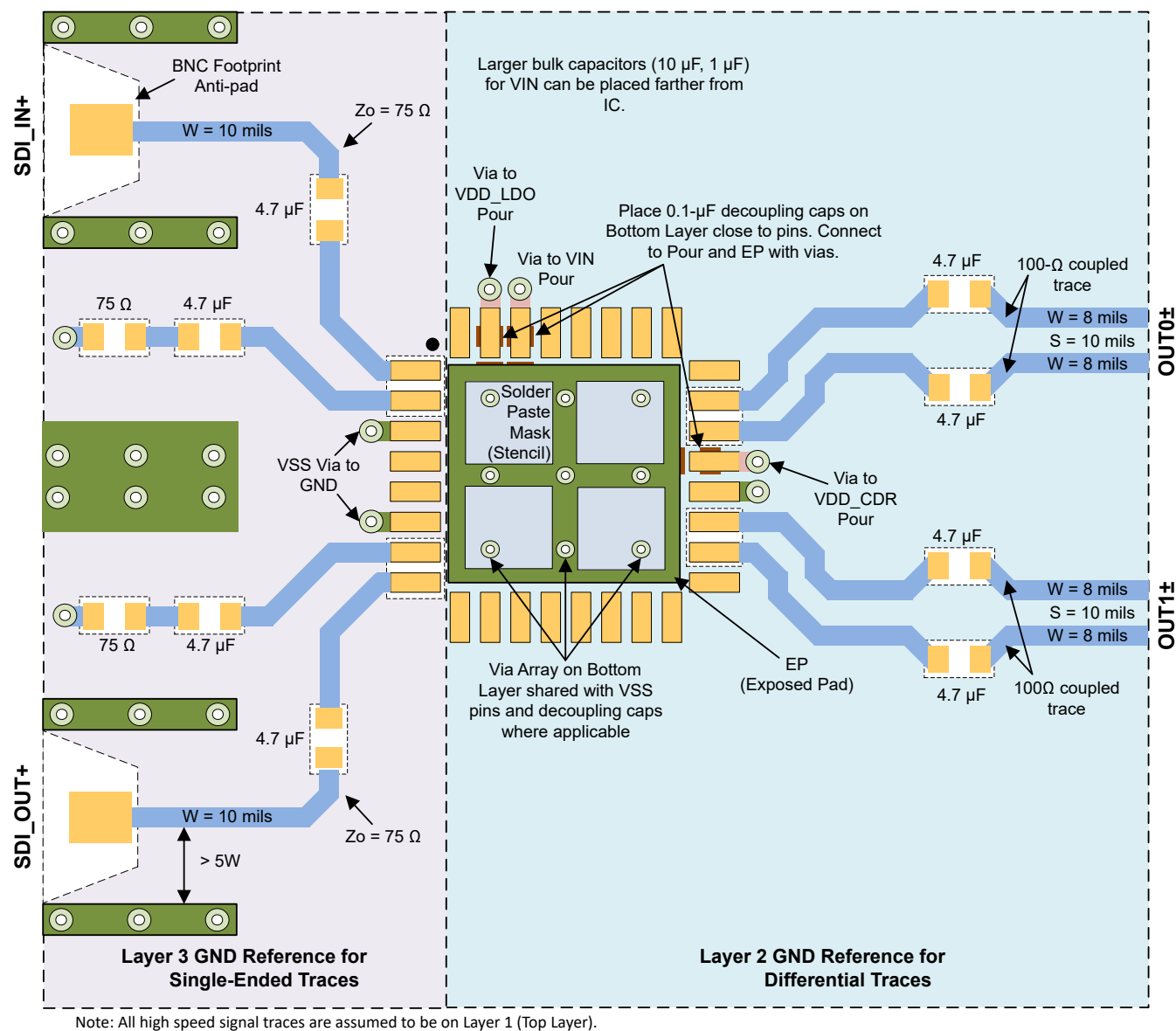
图 7-19. LMH12x9 高速布线布局示例
