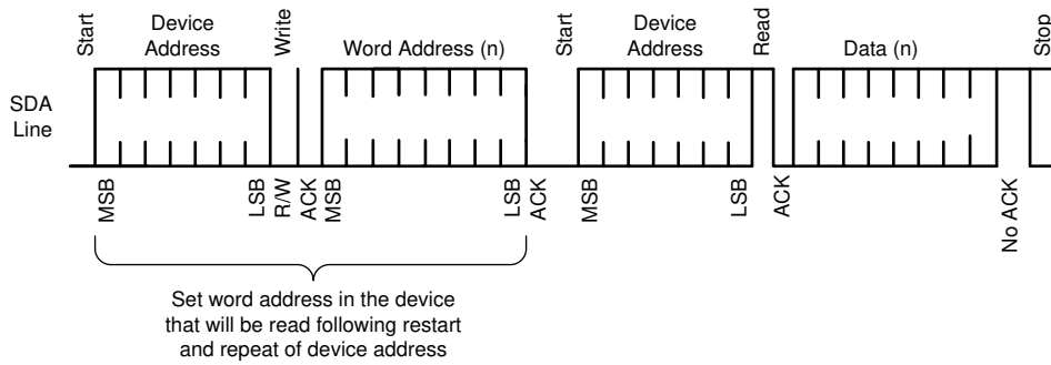
图 6-6. SMBus 读操作
