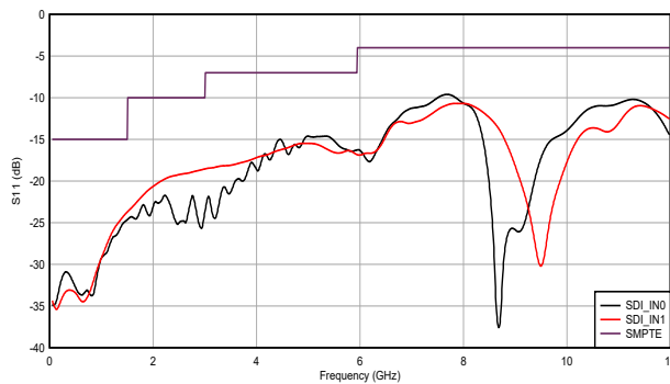
图 5-5. 输入回波损耗 (RL) 与频率间的关系
