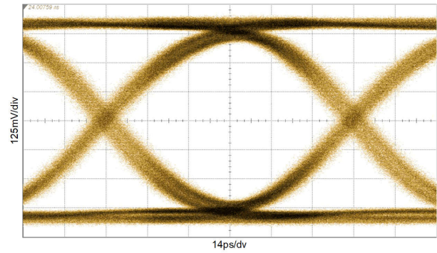
图 7-13. OUT0± 为 11.88Gbps (12G-SDI), CC = 100m Belden 1694A 位于 SDI_IN1+, 经过时钟恢复
