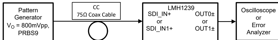
图 7-11. LMH12x9 PCB 输出及冗余 SDI 输入的测试设置
