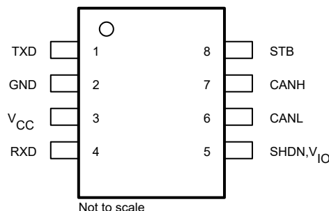
图 5-2. D Package, 8-Pin SOIC (Top View)
