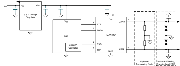
简化原理图
