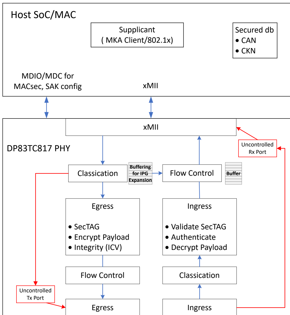
图 5-1. MACsec 方框图
