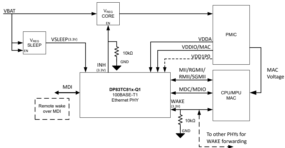
图 5-4. 系统方框图
