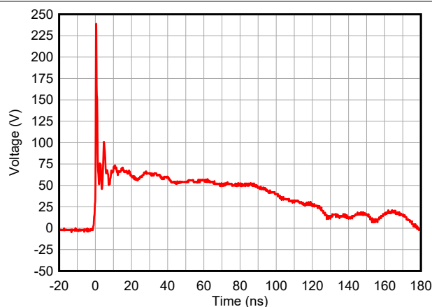
图 5-9. +8kV Clamped IEC Waveform
