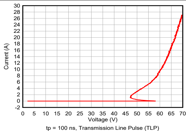
图 5-7. Positive TLP Curve
