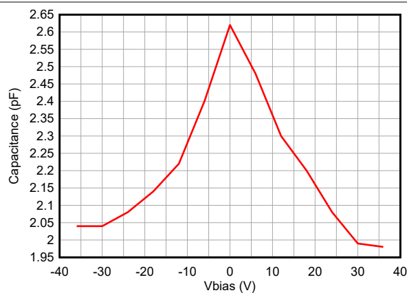
图 5-5. 电容与偏置电压之间的关系
