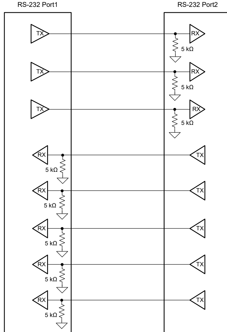
图 8-3. RS-232 serial communication
