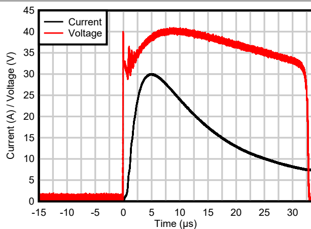
图 5-1. 8/20 \mu s 浪涌响应
