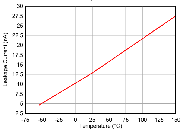
图 5-3. 漏电流与温度之间的关系
