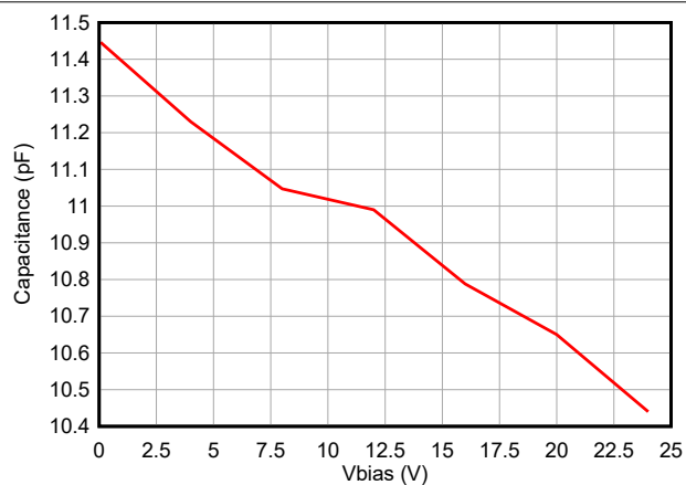
图 5-2. 电容与偏置电压之间的关系
