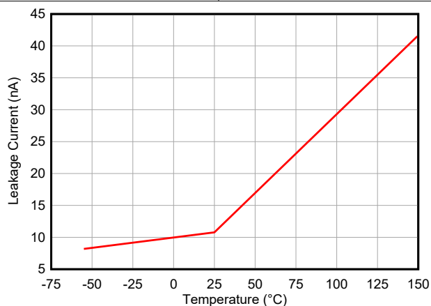
图 6-3. 漏电流与温度之间的关系
