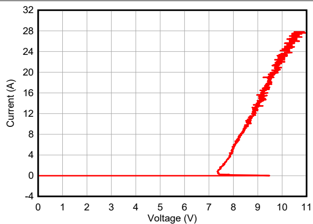
图 6-2. 负 TLP 曲线
