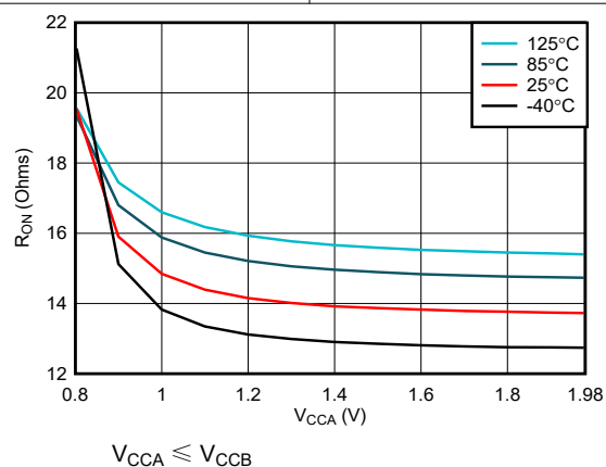
图 5-3. R_{ON} (Ω) vs \text{Min}(V_{CCA}, V_{CCB}) (V)
