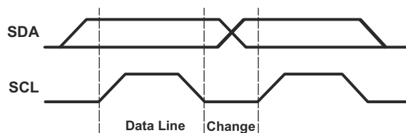
图 8-5. 位传输
