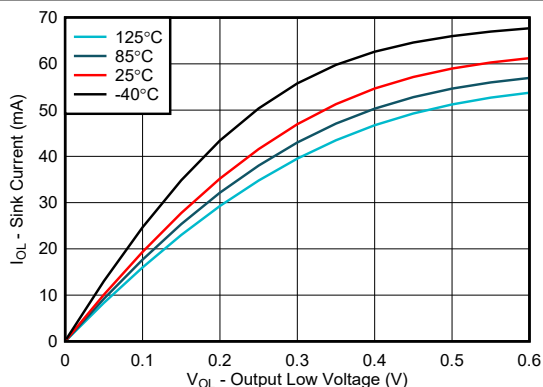
图 6-7. I/O 灌电流与输出低电压的关系, V_{CC} = 1.2\text{V}
