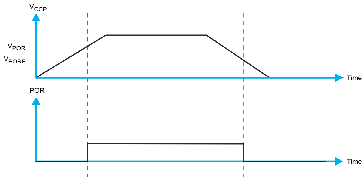
图 9-9. V_{POR}
