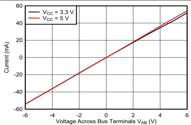
图 8-4. 终端开启时 AB 总线引脚上的电压与电流之间的关系
