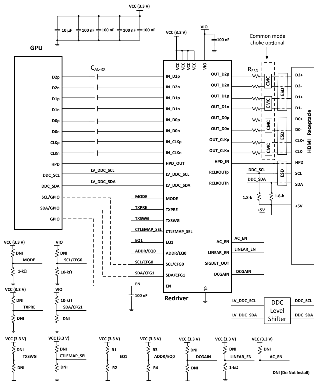
图 8-2. TMD51204 在源应用原理图
