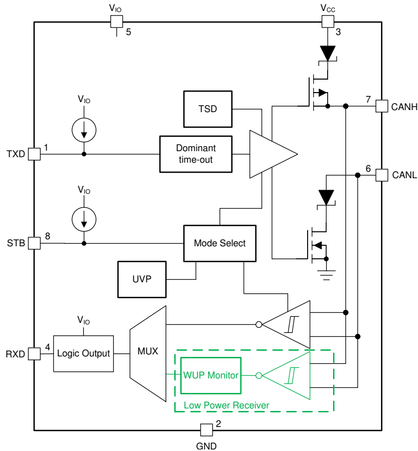
图 8-1. Block Diagram
