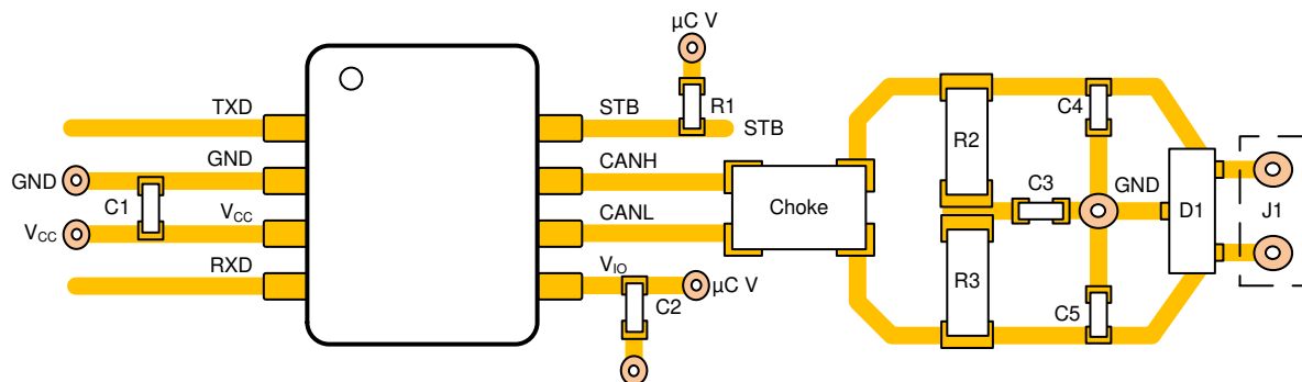
图 11-1. Layout Example
