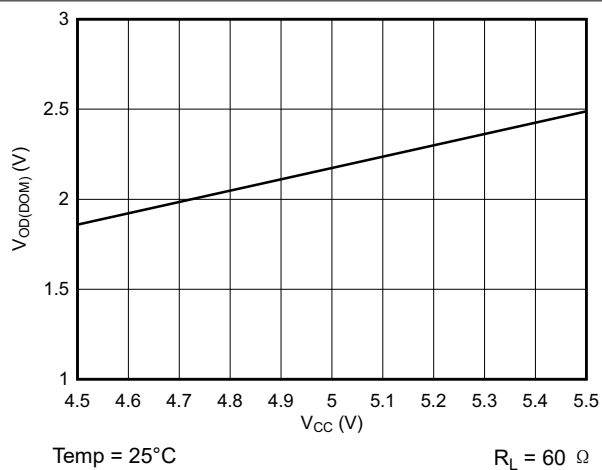
图 7-2. V_{OD(DOM)} vs V_{CC}
