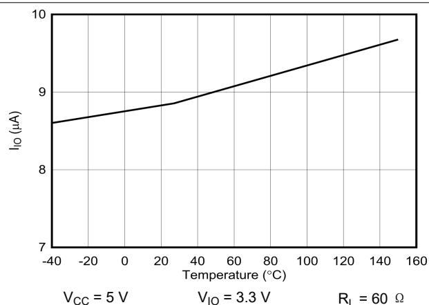
图 7-4. I_{IO} Standby vs Temperature
