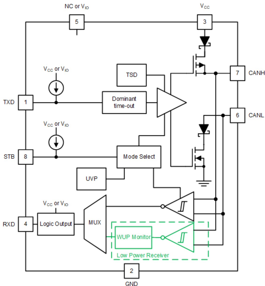
图 9-1. Block Diagram
