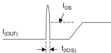
图 9-5. 输出短路参数
