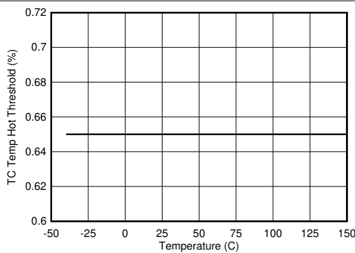
图 8-24. TS 高温阈值与结温之间的关系
