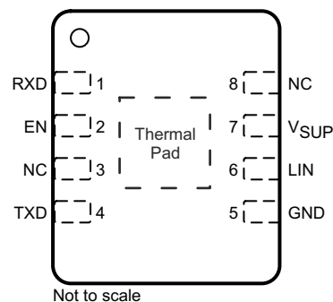
图 4-2. DRB Package, 8-Pin (VSON) (Top View)
