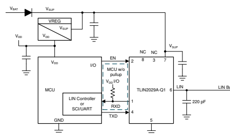
简化版原理图，响应者模式
