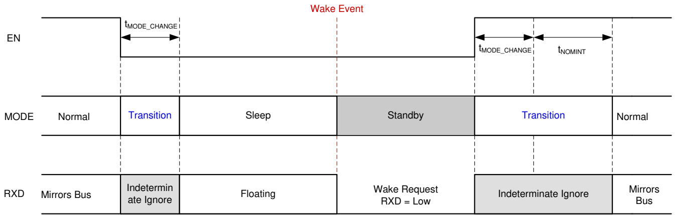
图 6-14. Mode Transitions
