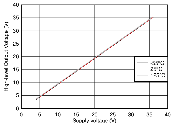
图 5-1. V_{OH} vs V_{SUP} and Temperature
