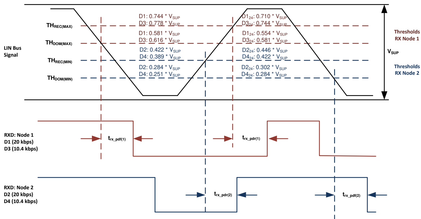
图 8-11. Propagation Delay
