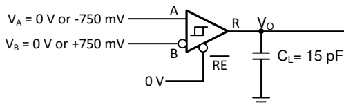
图 7-8. 驱动器被禁用情况下接收器启用次数的测量
