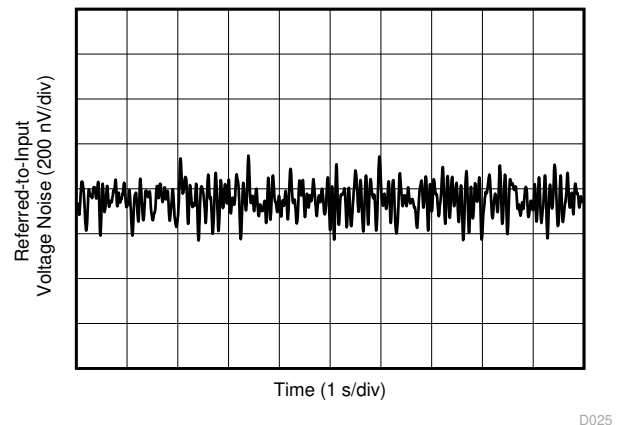
图 7-30. 0.1Hz 至 10Hz 电压噪声 (以输入为参考)
