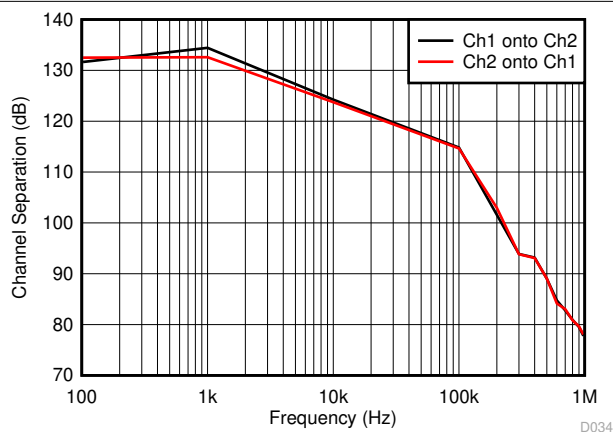
图 6-38. 通道分离与频率间的关系 (INA2181)
