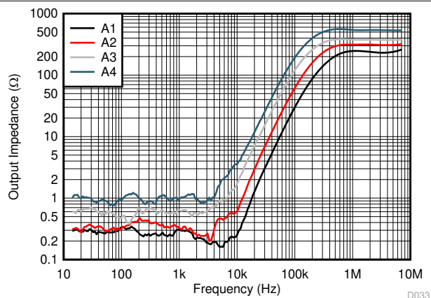
图 6-37. 输出阻抗与频率间的关系
