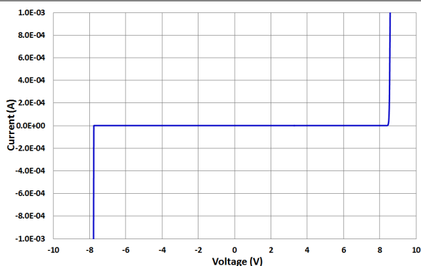
图 6-5. IV Curve
