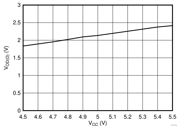
图 6-2. V_{OD(D)} over V_{CC}
