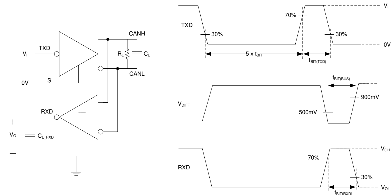
图 7-5. CAN FD Timing Parameter Measurement
