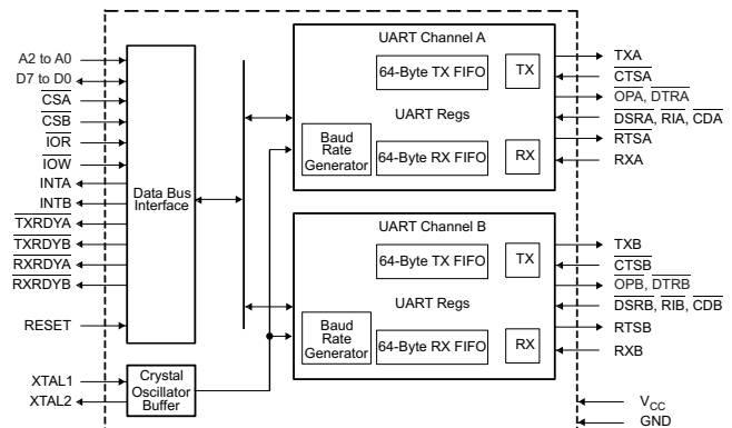
框图
