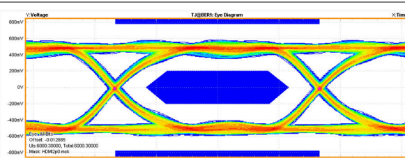
图 8-7. 6-Gbps HDMI 2.0 (TP1) Eye Diagram TPD1E05U06
