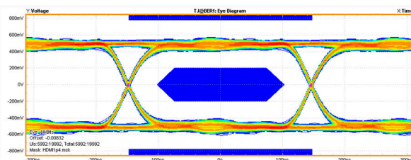
图 8-5. 3.4-Gbps HDMI 1.4 TP1 Eye Diagram TPD6E05U06
