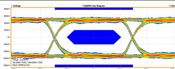
图 8-3. 3.4-Gbps HDMI 1.4 TP1 Eye Diagram TPD1E05U06
