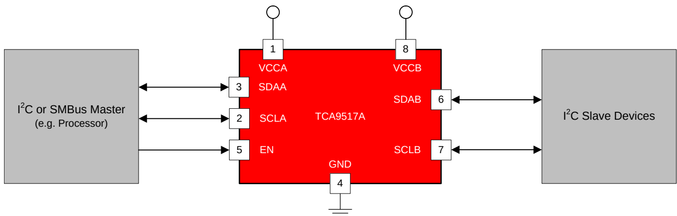
简化原理图
