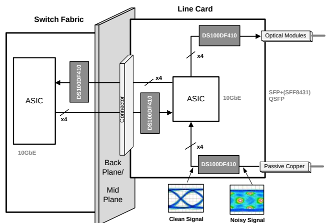
典型应用图
