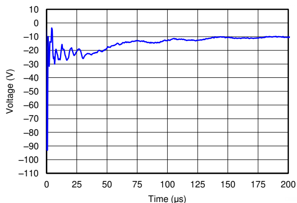
图 6-6. -8 kV IEC Waveform
