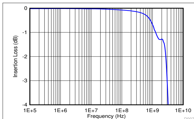
图 6-7. Insertion Loss
