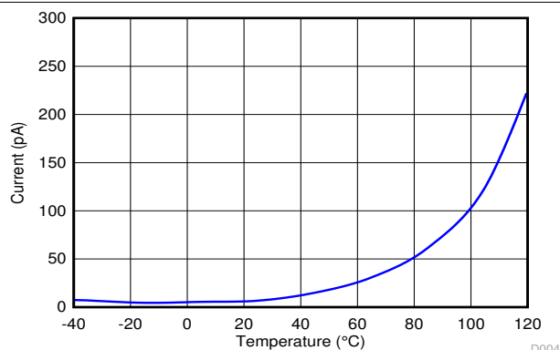
图 6-4. Leakage vs Temperature
