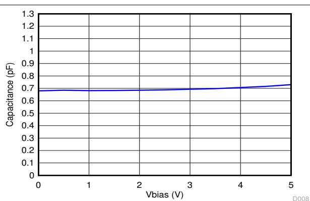
图 6-8. Capacitance vs V_{BIAS}
