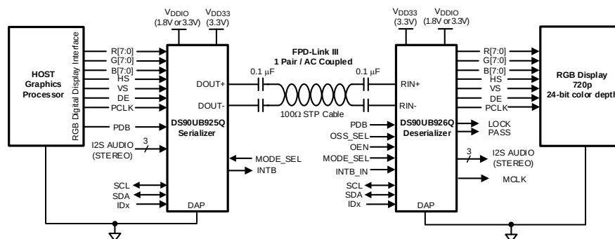
典型显示系统图
