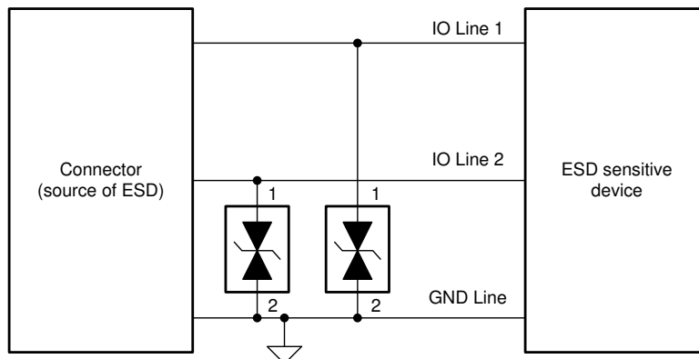
应用原理图
