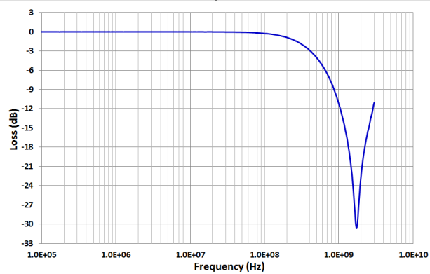
图 6-9. Insertion Loss
