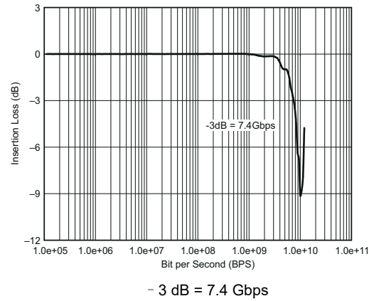
图 6-7. Insertion Loss
