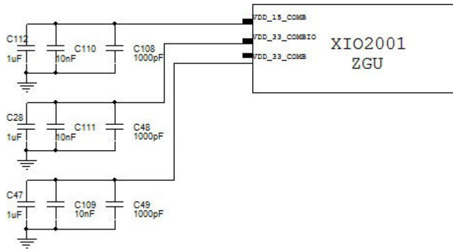
图 9-7. Combined Power
