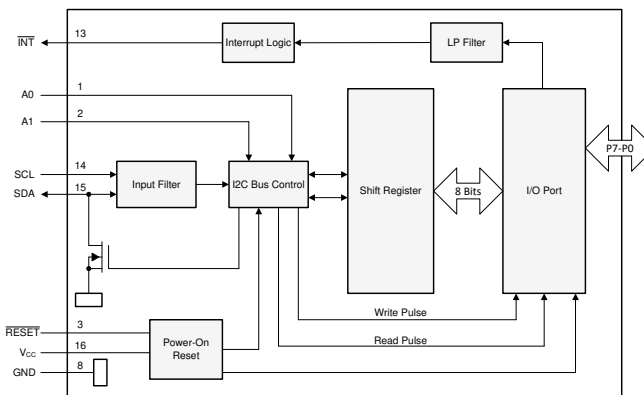
方框图
