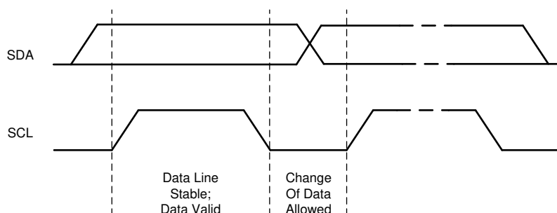
图 7-4. Bit Transfer
