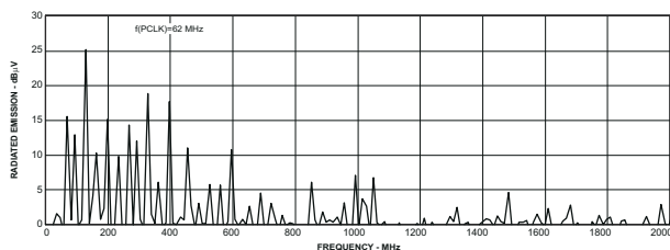
图 6-20. GTEM SAE J1752/3 EMI Test
