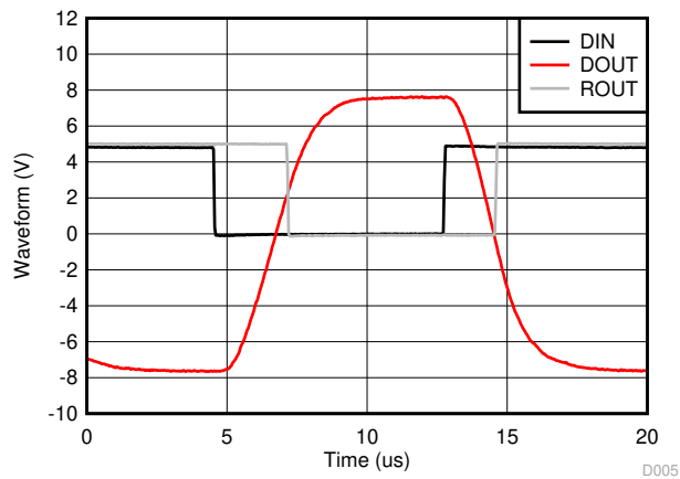
图 7-2. Loopback Waveforms
