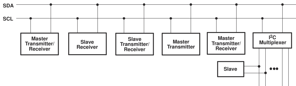
图 8-3. System Configuration
