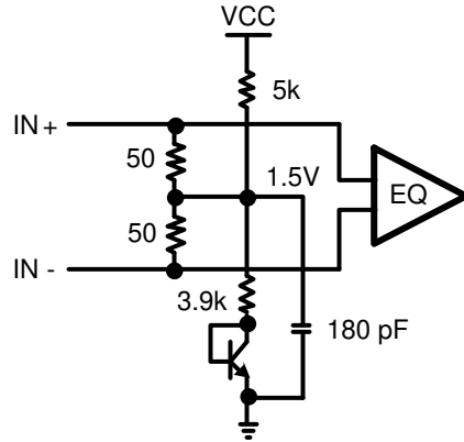
图 7-1. 接收器输入终端和偏置电路
