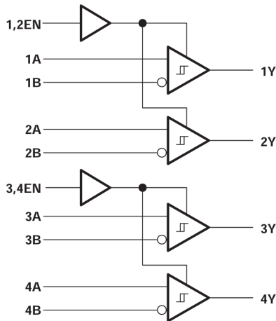
逻辑图 1
