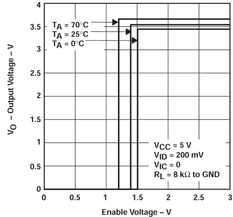
图 5-2. Output Voltage vs Enable Voltage
