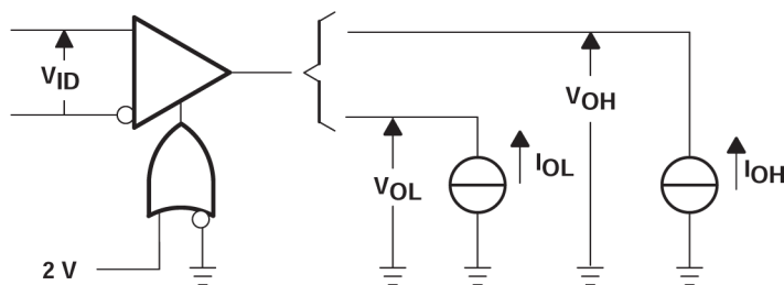
图 6-1. V_{OH} , V_{OL}
