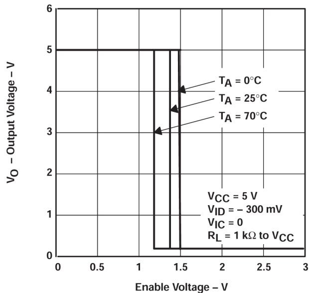
图 5-4. Output Voltage vs Enable Voltage
