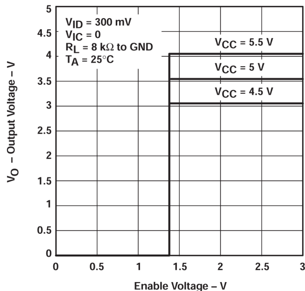
图 5-1. Output Voltage vs Enable Voltage
