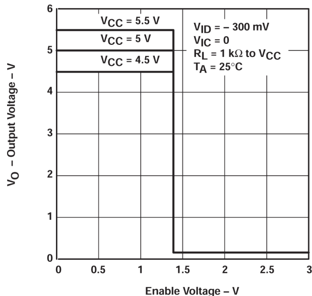
图 5-3. Output Voltage vs Enable Voltage
