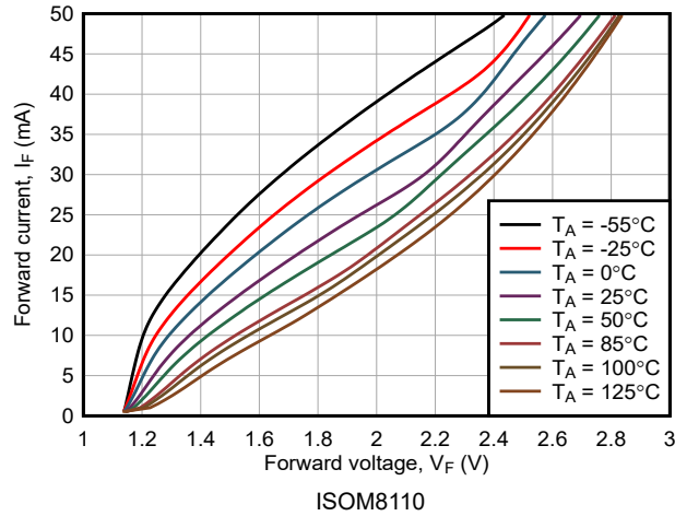
图 6-3. 正向电压与正向电流间的关系
