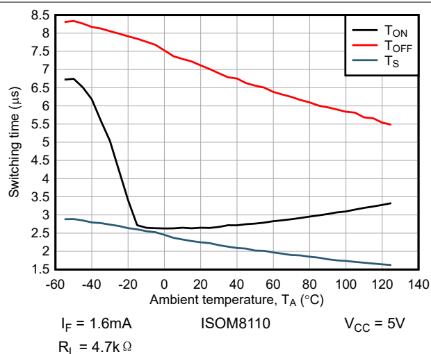
图 6-12. 开关时间与环境温度间的关系
