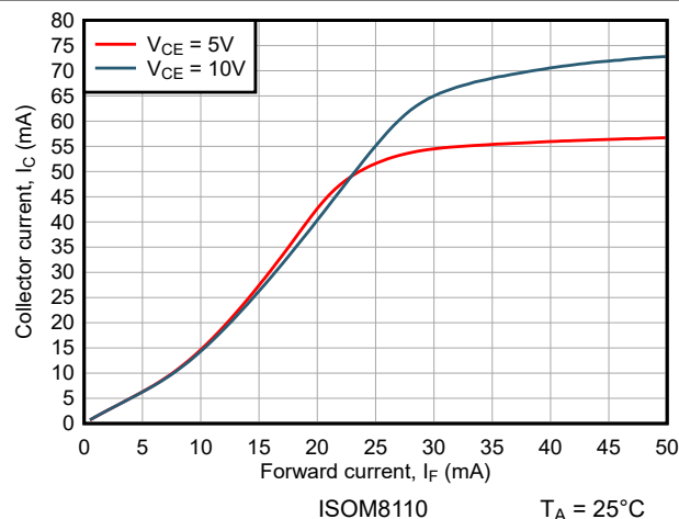
图 6-7. 集电极电流与正向电流间的关系
