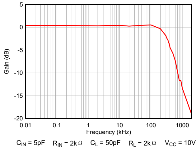
图 9-4. R_L = 2\text{k}\Omega 时的带宽
