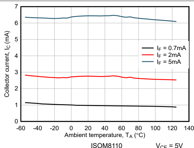
图 6-9. 集电极电流与环境温度间的关系
