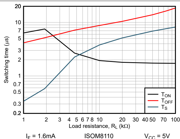
图 6-11. 开关时间与负载电阻间的关系
