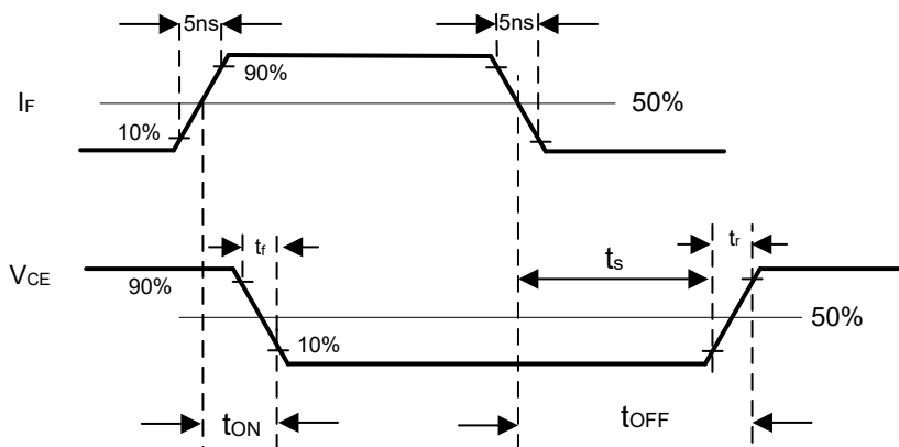
图 7-3. ISOM811x 开关时序波形
