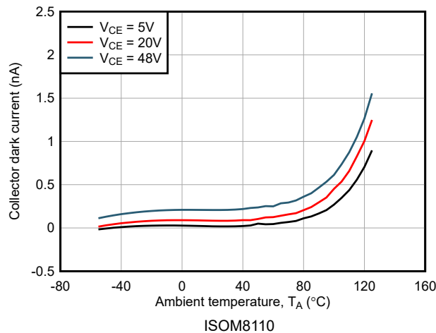
图 6-5. 集电极暗电流与环境温度间的关系
