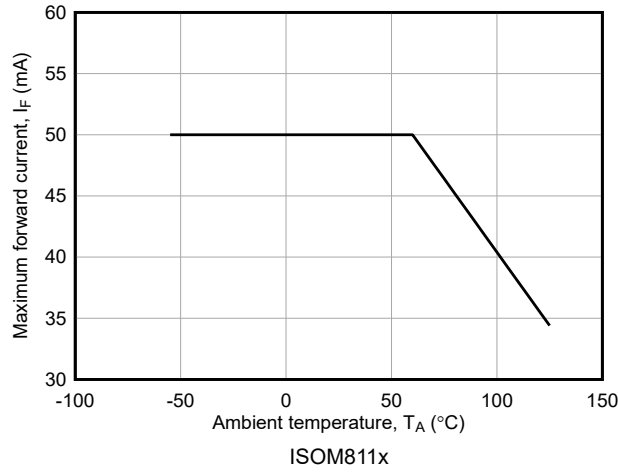
图 6-1. 最高正向电流与环境温度间的关系
