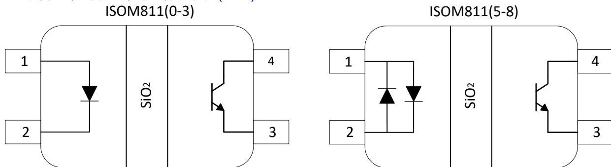
简化原理图
